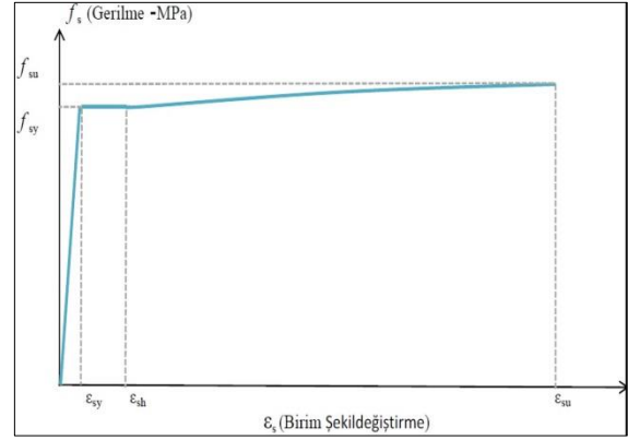
Şekil 2: Donatı malzeme modeli (Model pf material outfit)
