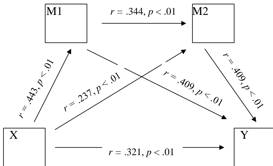
Figür 3.3.1.: Çoklu Arabuluculuk Modelinin İki Aracılı Değişkenli İstatiksel Diyagram
